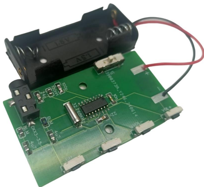
Мини FM радио с питанием от батареек
