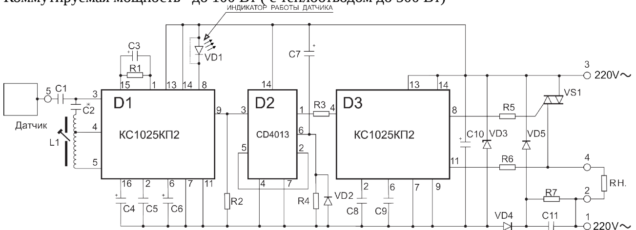
Рисунок 1. Принципиальная схема
