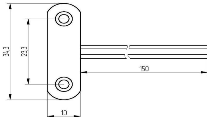
Рис.1. Габаритные и установочные размеры
