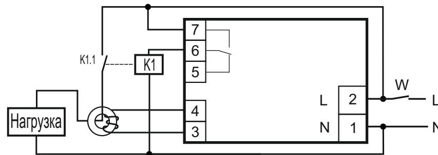
Рис.2. Схема подключения нагрузки к устройству RN 1F-73
