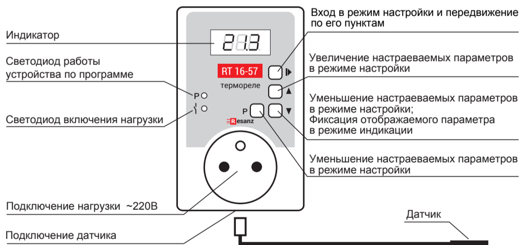
Рис. 1: устройство прибора
