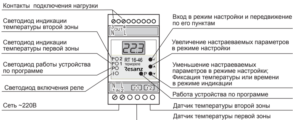
Рис. 1: устройство прибора
