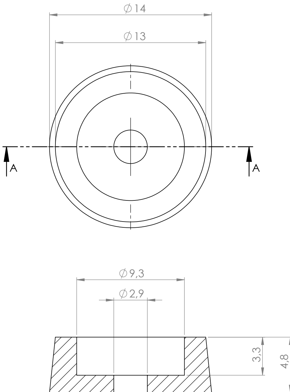
PRZEKRÓJ A-A SKALA 5 : 1
