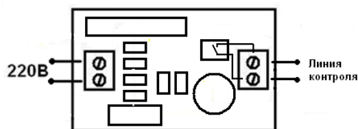
Схема подключения. Рис. 2
