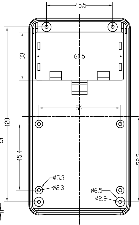
下盖正视图
