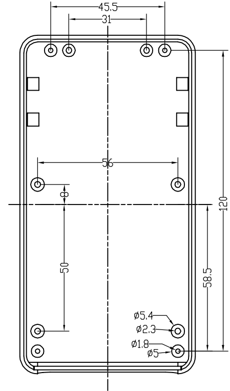
上盖底视图
