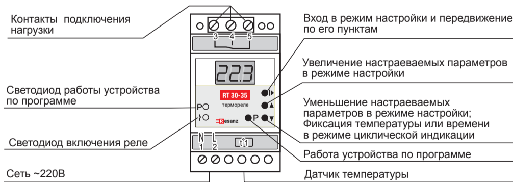
Рис. 1: устройство прибора
