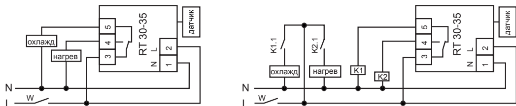
Рис. 2: схема подключения нагрузки мощностью до 4,4 кВт к устройству
