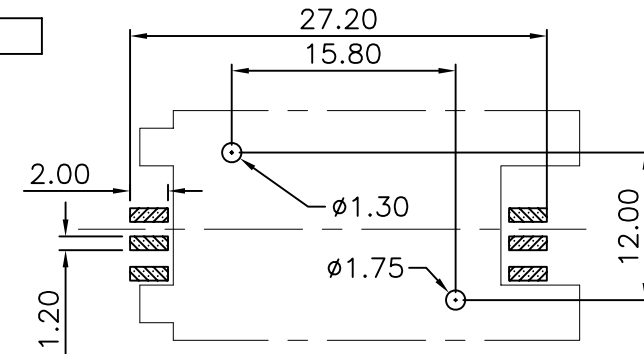
P.C.B. Layout
